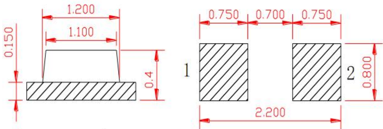
焊盘图
